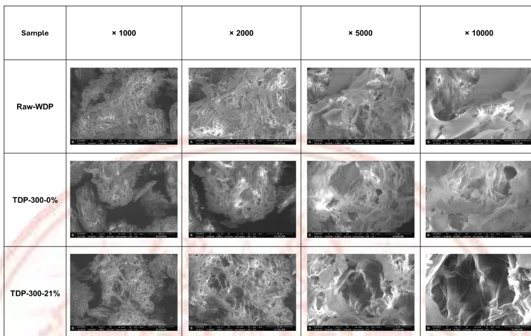
ภาพที่ 4-19 การวิเคราะห์ลักษณะทางกายภาพของเปลือกทุเรียนและผลิตภัณฑ์ทอรรีไฟด์เปลือกทุเรียนที่ผ่านการล้างด้วยน้ำ ที่อุณหภูมิ 300 °C ระยะเวลาที่คงอยู่ในเครื่องปฏิกรณ์ 30 นาที ภายใต้สภาวะออกซิเจนร้อยละ 0 และ 21
