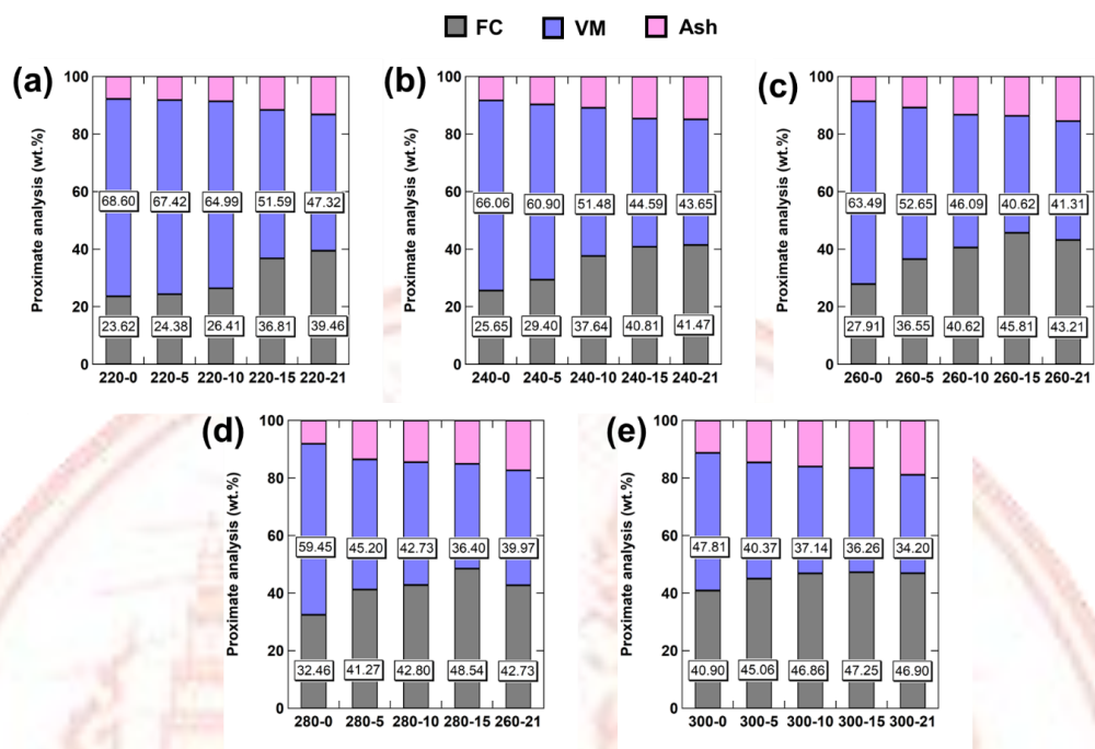
ภาพที่ 4-8 การวิเคราะห์แบบประมาณของผลิตภัณฑ์ทอร์รีไฟด์เปลือกทุเรียนที่อุณหภูมิ (a) 220 °C (b) 240 °C (c) 260 °C (d) 280 °C และ (e) 300 °C ระยะเวลาที่คงอยู่ในเครื่องปฏิกรณ์ 30 นาที ภายใต้สภาวะออกซิเจนต่าง ๆ
