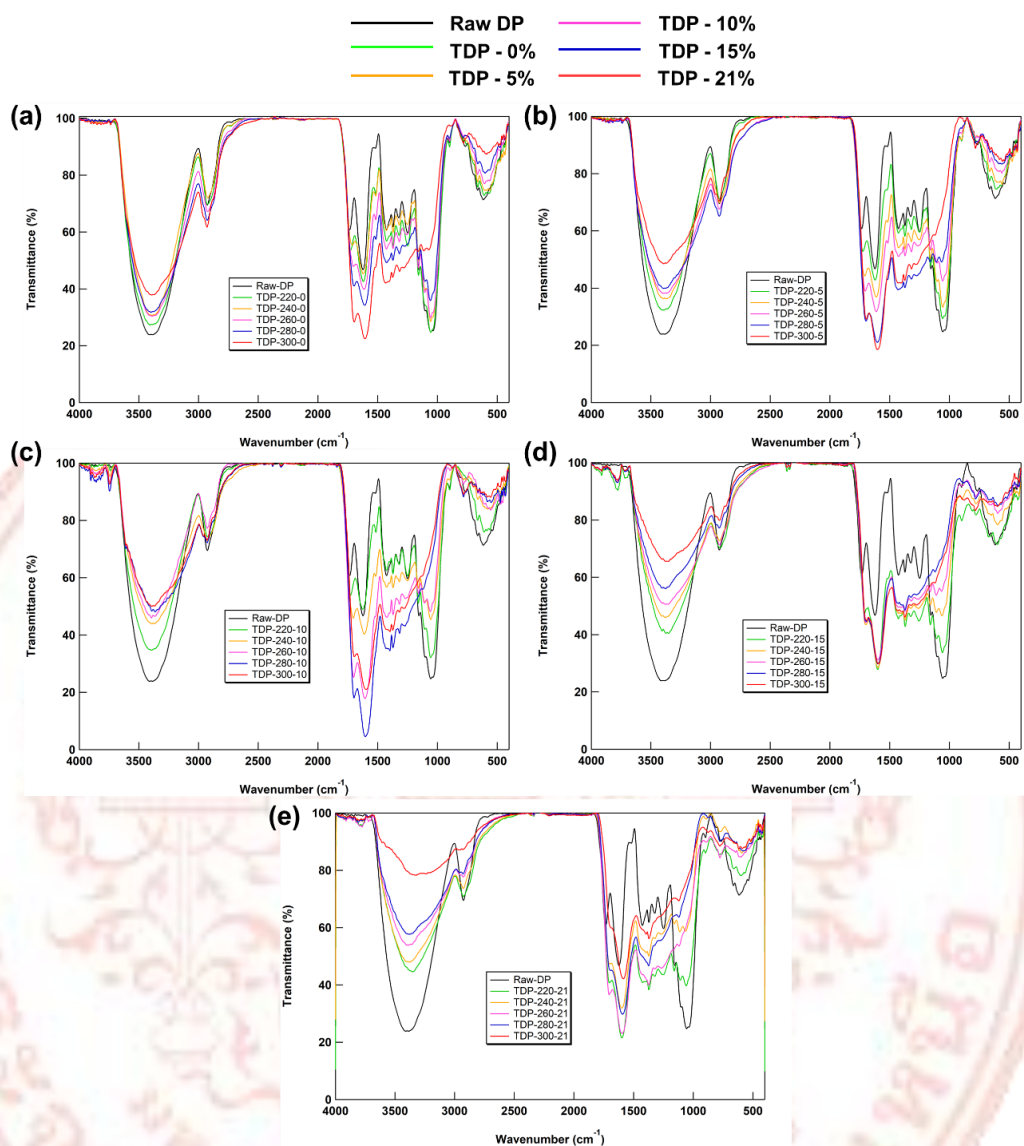
ภาพที่ 4-17 การวิเคราะห์หมู่ฟังก์ชันของผลิตภัณฑ์ทอร์รีไฟด์เปลือกทุเรียนที่ปริมาณความเข้มข้นออกซิเจน (a) ร้อยละ 0 (b) ร้อยละ 5 (c) ร้อยละ 10 (d) ร้อยละ 15 และ (e) ร้อยละ 21 ภายใต้สภาวะอุณหภูมิต่าง ๆ
