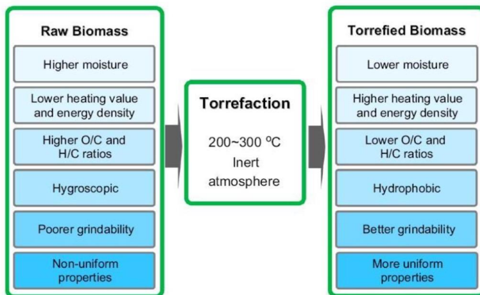
ภาพที่ 2-4 สมบัติของชีวมวลก่อนและกระบวนการทอร์รีแฟกชัน
