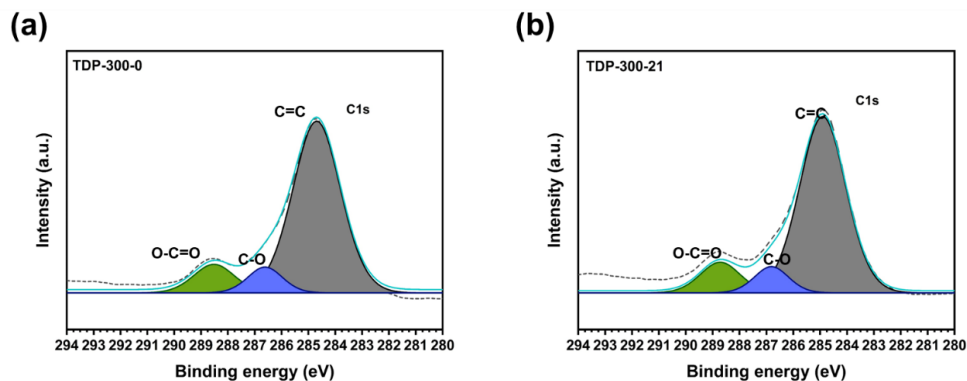
ภาพที่ 4-24 สเปกตรัม XPS ของผลิตภัณฑ์ทอร์รีไฟด์เปลือกทุเรียนในย่านพลังงานของ C1s
