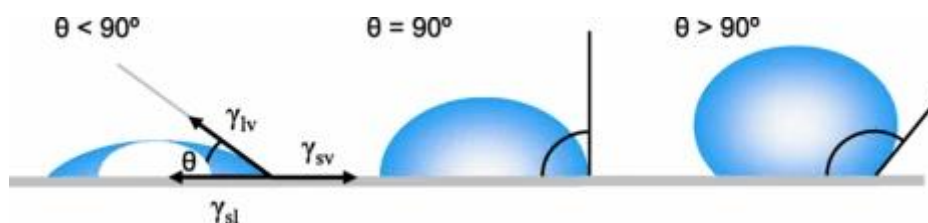
ภาพที่ 2-8 มุมสัมผัสสามารถจำแนกสมบัติของวัสดุ [45]
