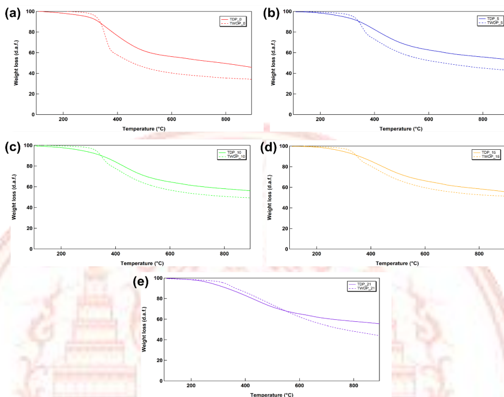
ภาพที่ 4-22 การสลายตัวทางความร้อนของของผลิตภัณฑ์เทอร์รีไฟด์เปลือกทุเรียนที่ไม่ผ่านการล้างด้วยน้ำและล้างด้วยน้ำ (a) 220 °C (b) 240 °C (c) 260 °C (d) 280 °C และ (e) 300 °C ระยะเวลาที่คงอยู่ในเครื่องปฏิกรณ์ 30 นาที ภายใต้สภาวะออกซิเจนต่างๆ
