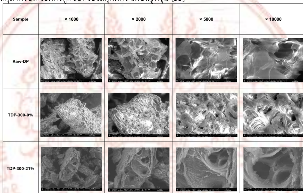
ภาพที่ 4-3 การวิเคราะห์ลักษณะทางกายภาพของเปลือกทุเรียนและผลิตภัณฑ์ทอรรีไฟต์เปลือกทุเรียนที่อุณหภูมิ 300 °C ระยะเวลาที่คงอยู่ในเครื่องปฏิกรณ์ 30 นาที ภายใต้สภาวะออกซิเจนร้อยละ 0 และ 21
