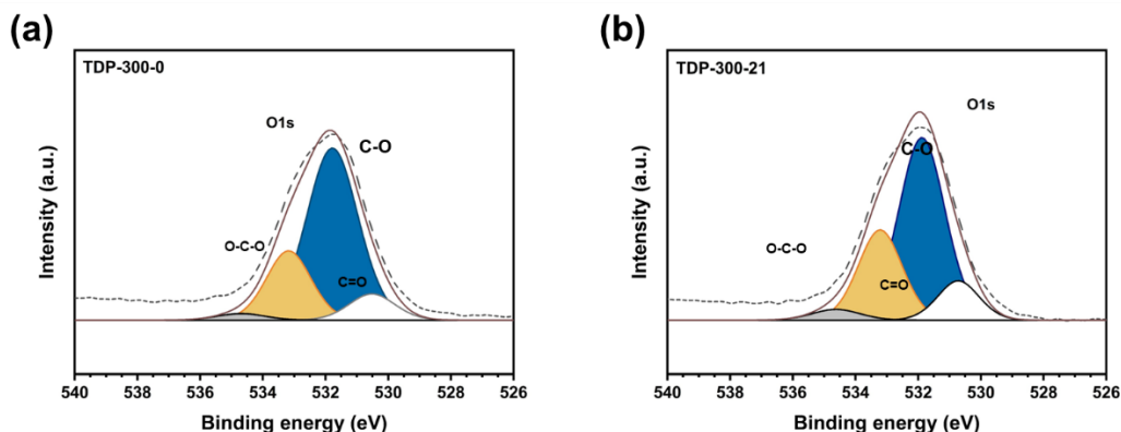
ภาพที่ 4-26 สเปกตรัม XPS ของผลิตภัณฑ์ทอร์รีไฟด์เปลือกทุเรียนในย่านพลังงานของ O1s
