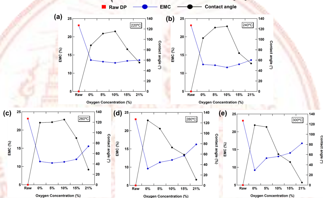
ภาพที่ 4-14 ความสัมพันธ์ของการวิเคราะห์ความชื้นสมดุลและมัมสัมพัทธ์ของผลิตภัณฑ์ทอร์รีไฟด์ เปลือกทุเรียนที่อุณหภูมิ (a) 220 °C (b) 240 °C (c) 260 °C (d) 280 °C และ (e) 300 °C ระยะเวลาที่คงอยู่ในเครื่องปฏิกรณ์ 30 นาที ภายใต้สภาวะออกซิเจนต่าง ๆ
