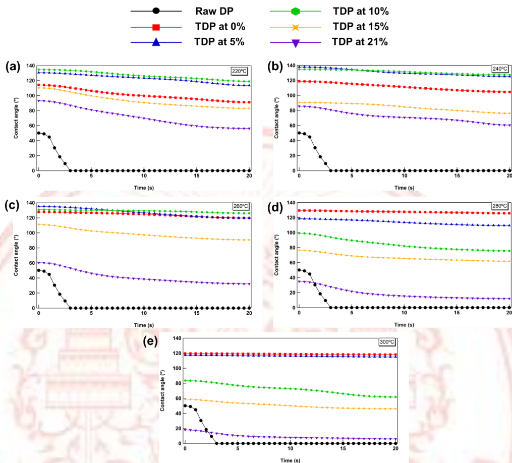
ภาพที่ 4-10 การวิเคราะห์มุมสัมผัสของผลิตภัณฑ์ทอรรีไฟด์เปลือกทุเรียนที่อุณหภูมิ (a) 220 °C (b) 240 °C (c) 260 °C (d) 280 °C และ (e) 300 °C ระยะเวลาที่คงอยู่ในเครื่องปฏิกรณ์ 30 นาที ภายใต้สภาวะออกซิเจนต่าง
