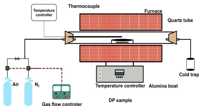
ภาพที่ 3-1 Torrefaction Horizontal Tube Reactor
