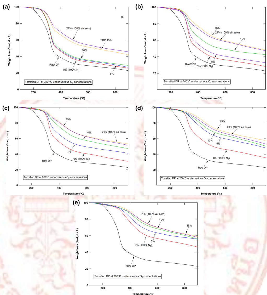
ภาพที่ 4-7 การสลายตัวทางความร้อนของผลิตภัณฑ์ทอร์รีไฟด์เปลือกทุเรียนที่อุณหภูมิ (a) 220 °C (b) 240 °C (c) 260 °C (d) 280 °C และ (e) 300 °C ระยะเวลาที่คงอยู่ในเครื่องปฏิกรณ์ 30 นาที ภายใต้สภาวะออกซิเจนต่างๆ
