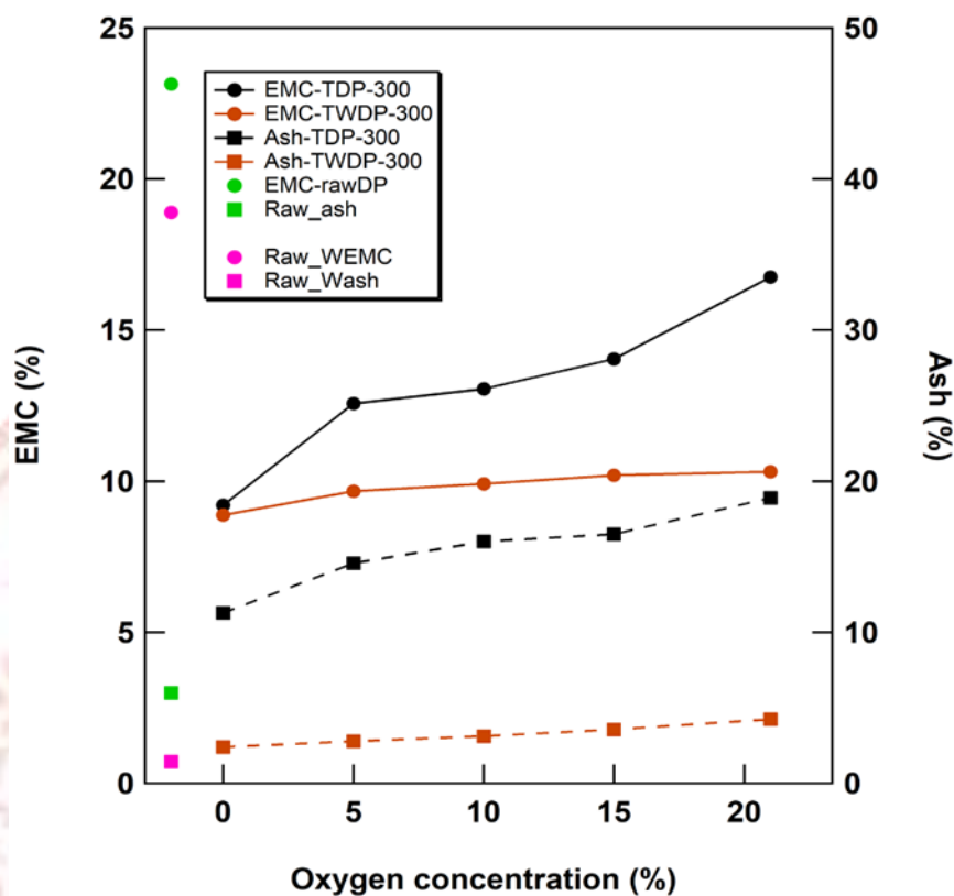
ภาพที่ 4-31 ความสัมพันธ์ของการวิเคราะห์ความชื้นสมดุลและปริมาณเถ้าของผลิตภัณฑ์เทอร์รี่ไฟต์ เปลือกทุเรียนที่ก่อนและหลังล้างน้ำที่ 300 °C ระยะเวลาที่คงอยู่ในเครื่องปฏิกรณ์ 30 นาที ภายใต้สภาวะออกซิเจนต่าง ๆ
