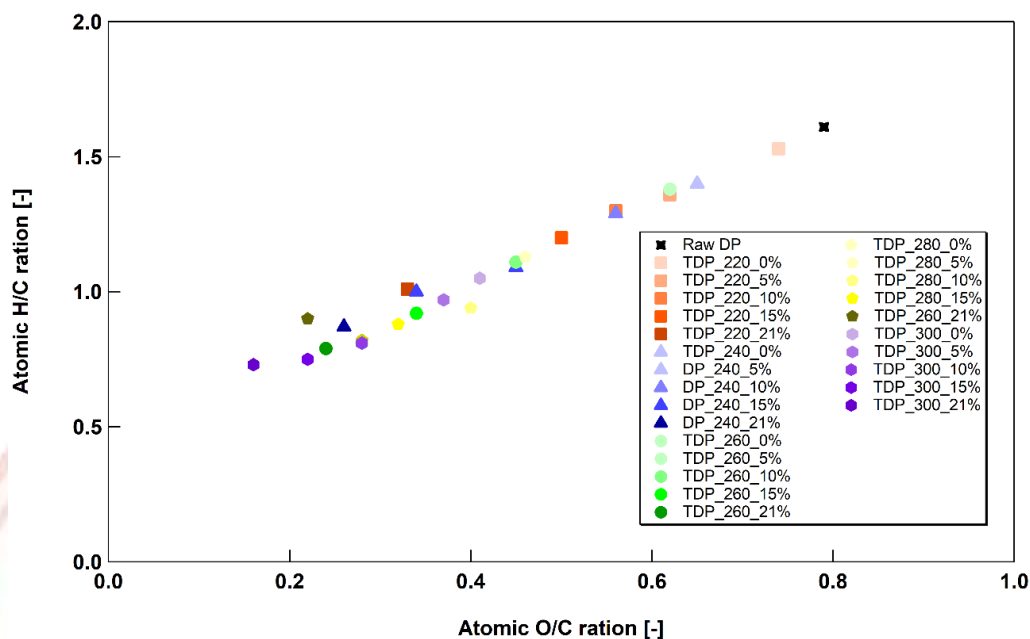
ภาพที่ 4-6 แผนภาพ Van Krevelen ของผลิตภัณฑ์ทอร์รีไฟด์เปลือกทุเรียนที่อุณหภูมิ 220 - 300 °C ระยะเวลาที่คงอยู่ในเครื่องปฏิกรณ์ 30 นาที ภายใต้สภาวะออกซิเจนต่างๆ
