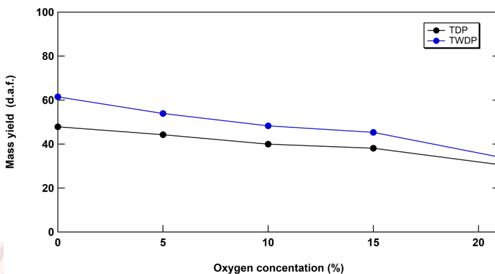
ภาพที่ 4-18 ความสัมพันธ์ของร้อยละผลได้เชิงมวลของผลิตภัณฑ์ทอร์รีไฟด์เปลือกทุเรียนที่ไม่ผ่านการล้างด้วยน้ำและล้างด้วยน้ำ ที่อุณหภูมิ 300 °C ระยะเวลาที่คงอยู่ในเครื่องปฏิกรณ์ 30 นาที ภายใต้สภาวะออกซิเจนต่าง ๆ
