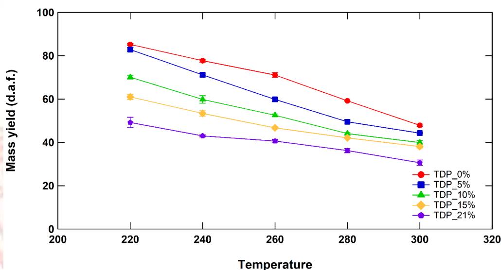
ภาพที่ 4-2 ร้อยละผลได้เชิงมวลของผลิตภัณฑ์ทอร์รีไฟด์เปลือกทุเรียนที่อุณหภูมิ 220 - 300 °C ระยะเวลาที่คงอยู่ในเครื่องปฏิกรณ์ 30 นาที ภายใต้สภาวะออกซิเจนต่างๆ
