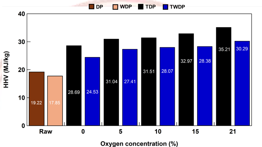
ภาพที่ 4-21 ความสัมพันธ์ของค่าความร้อนสูงสุดของผลิตภัณฑ์ทอร์รีไฟต์เปลือกทุเรียนที่ไม่ผ่านการล้างด้วยน้ำและล้างด้วยน้ำ ที่อุณหภูมิ 300 °C ระยะเวลาที่คงอยู่ในเครื่องปฏิกรณ์ 30 นาที ภายใต้สภาวะออกซิเจนต่าง ๆ
