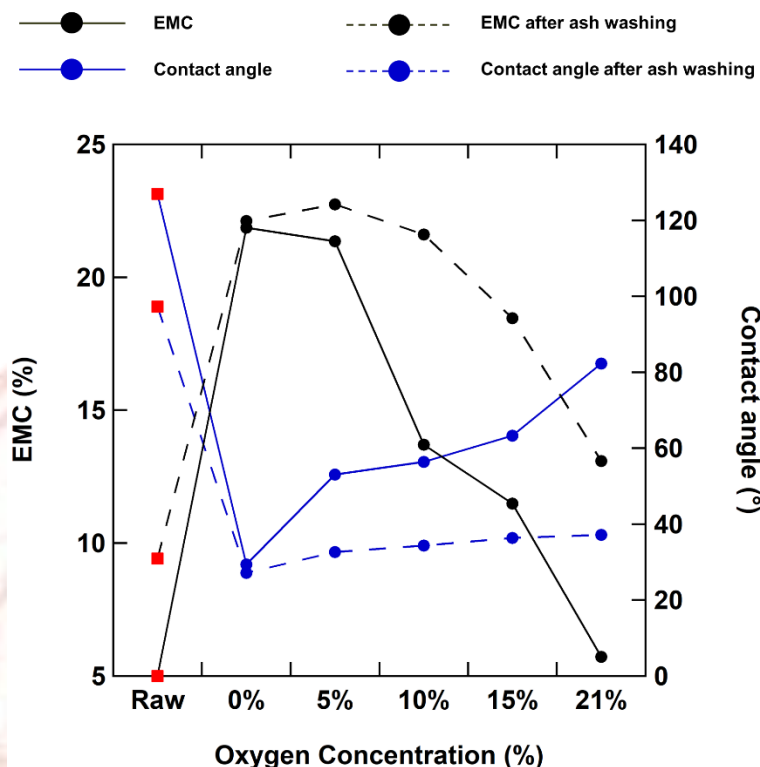
ภาพที่ 4-30 ความสัมพันธ์ของการวิเคราะห์ความชื้นสมดุลและมุมสัมผัสของผลิตภัณฑ์ทอรรีไฟต์ เปลือกทุเรียนก่อนและหลังล้างน้ำที่ 300 °C ระยะเวลาที่คงอยู่ในเครื่องปฏิกรณ์ 30 นาที ภายใต้สภาวะออกซิเจนต่าง ๆ
