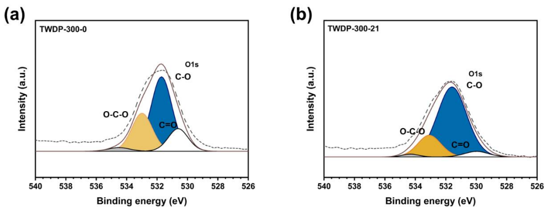
ภาพที่ 4-27 สเปกตรัม XPS ของผลิตภัณฑ์ทอร์รีไฟด์เปลือกทุเรียนในย่านพลังงานของ O1s
