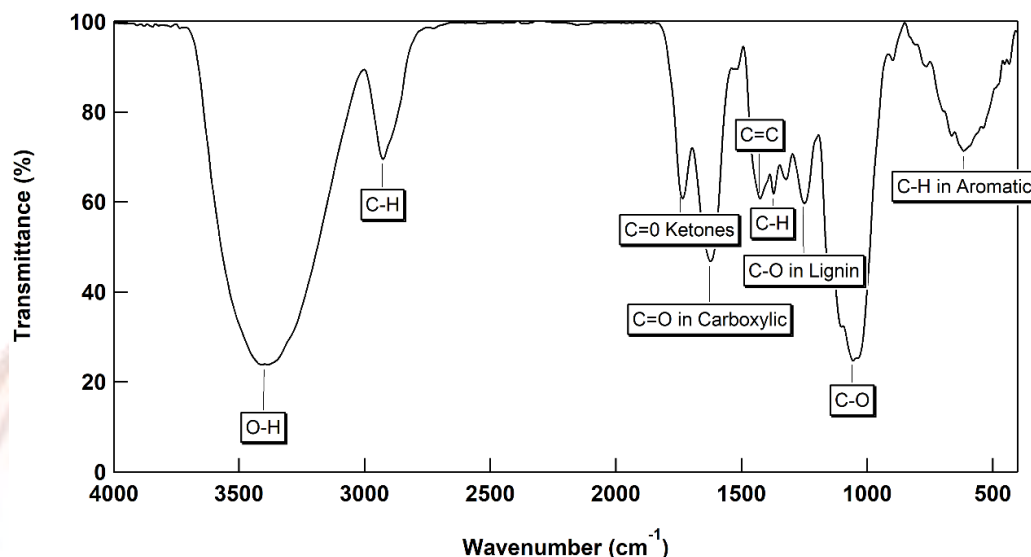
ภาพที่ 4-15 การวิเคราะห์หมู่ฟังก์ชันของเปลือกทุเรียนที่ไม่ผ่านกระบวนการออกซิเดทีฟเทอร์รีแฟกชัน
