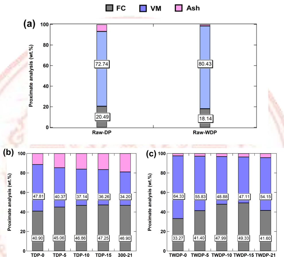
ภาพที่ 4-23 การวิเคราะห์แบบประมาณ (a) เปลือกทุเรียน (b) ผลิตภัณฑ์เทอร์รีไฟด์เปลือกทุเรียนที่ไม่ผ่านการล้างด้วยน้ำ (c) ผลิตภัณฑ์เทอร์รีไฟด์เปลือกทุเรียนที่ล้างด้วยน้ำ ที่อุณหภูมิ 300 °C ระยะเวลาที่คงอยู่ในเครื่องปฏิกรณ์ 30 นาที ภายใต้สภาวะออกซิเจนต่าง ๆ
