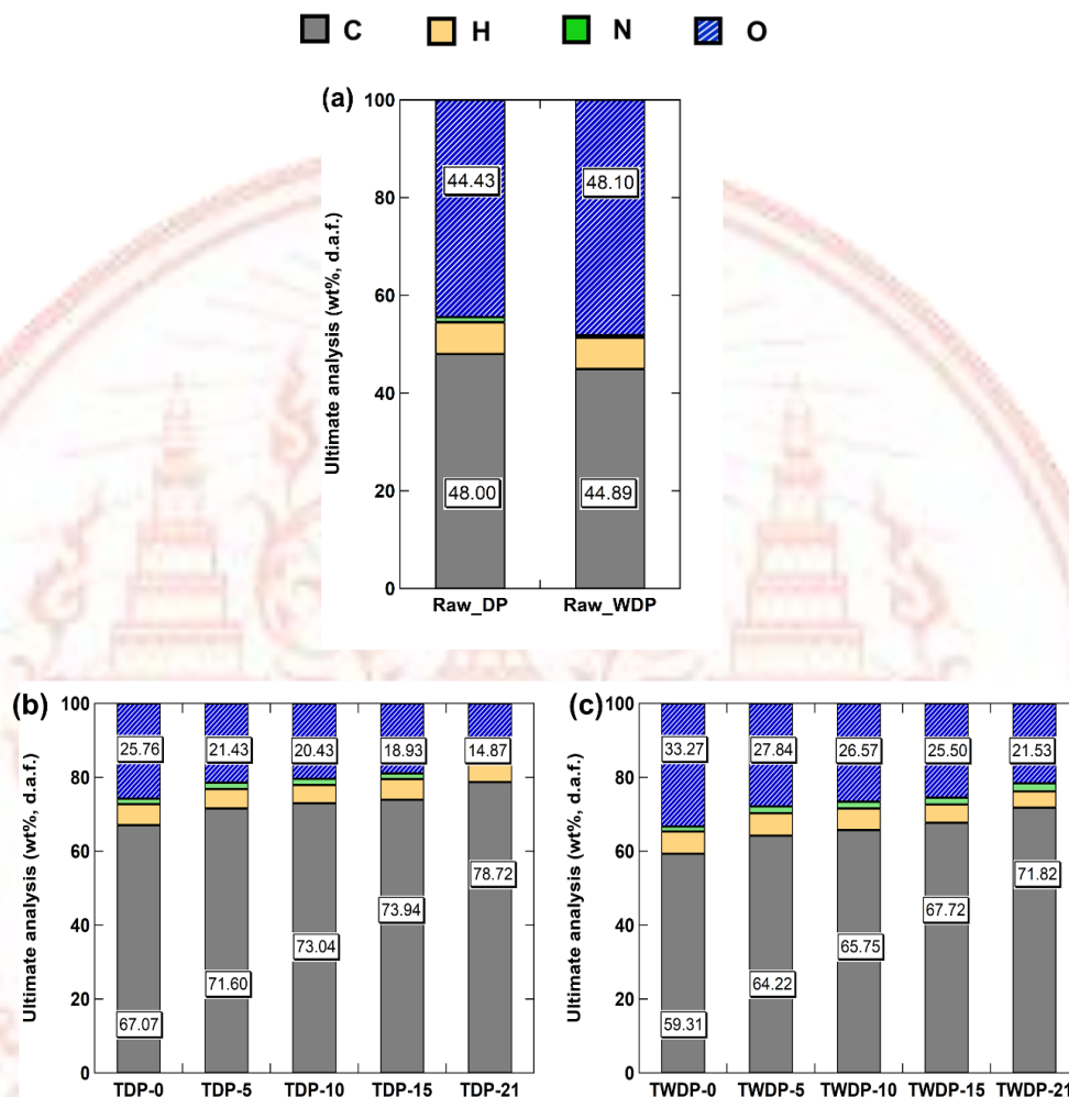
ภาพที่ 4-20 ปริมาณองค์ประกอบของ (a) เปลือกทุเรียน (b) ผลิตภัณฑ์ทอร์รีไฟด์เปลือกทุเรียนที่ไม่ผ่านการล้างด้วยน้ำ (c) ผลิตภัณฑ์ทอร์รีไฟด์เปลือกทุเรียนที่ล้างด้วยน้ำ ที่อุณหภูมิ 300 °C ระยะเวลาที่คงอยู่ในเครื่องปฏิกรณ์ 30 นาที ภายใต้สภาวะออกซิเจนต่าง ๆ
