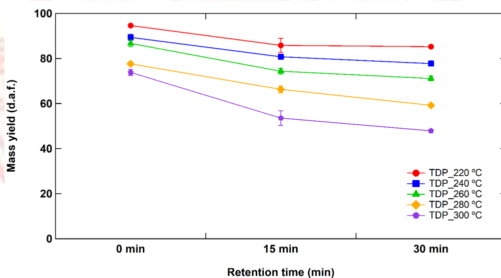
ภาพที่ 4-1 ร้อยละผลได้เชิงมวลของผลิตภัณฑ์ทอรรีไฟด์เปลือกทุเรียนที่อุณหภูมิ 220 - 300 °C ระยะเวลาที่คงอยู่ในเครื่องปฏิกรณ์ 0 15 และ 30 นาที ภายใต้สถานะไนโตรเจน
