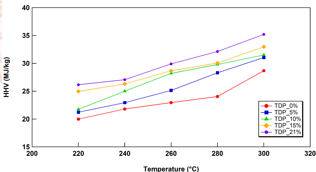
ภาพที่ 4-5 ค่าความร้อนสูงสุดของผลิตภัณฑ์ทอรรีไฟด์เปลือกทุเรียนที่อุณหภูมิ 220 - 300 °C ระยะเวลาที่คงอยู่ในเครื่องปฏิกรณ์ 30 นาที ภายใต้สภาวะออกซิเจนต่างๆ
