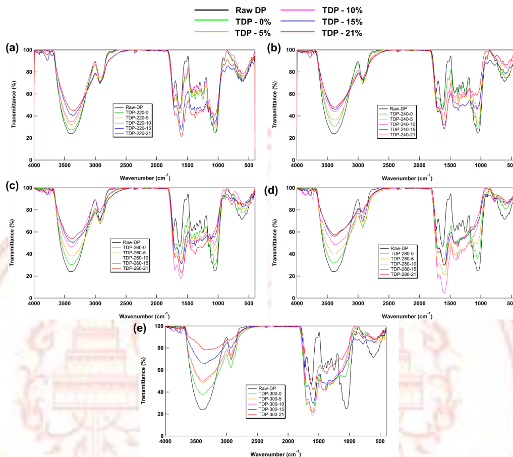
ภาพที่ 4-16 การวิเคราะห์หมู่ฟังก์ชันของผลิตภัณฑ์พอลิไทโอฟีนที่เลือกทุเรียนที่อุณหภูมิ (a) 220 °C (b) 240 °C (c) 260 °C (d) 280 °C และ (e) 300 °C ระยะเวลาที่คงอยู่ในเครื่องปฏิกรณ์ 30 นาที ภายใต้สภาวะออกซิเจนต่าง ๆ
