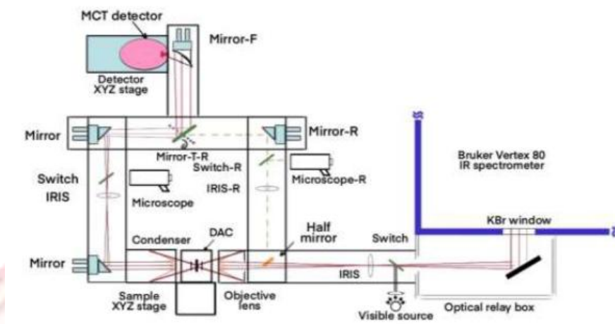
ภาพที่ 2-6 หลักการทำงานของเครื่องฟูเรียร์ทรานส์ฟอร์มอินฟราเรดสเปกโทรสโกปี [42]
