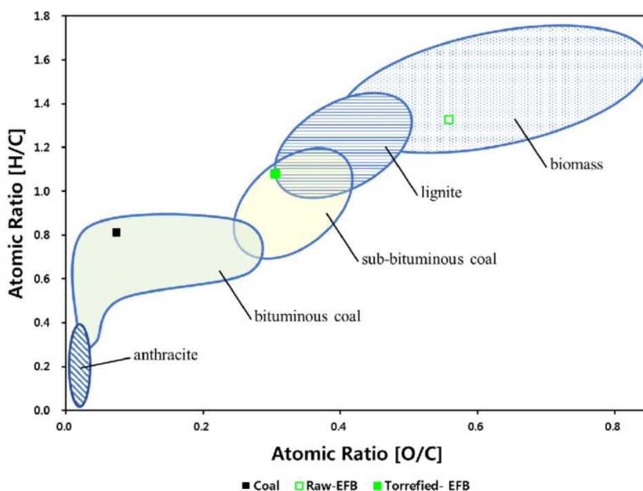
ภาพที่ 2-5 แผนภาพ Van Krevelen ของถ่านหิน [41]
