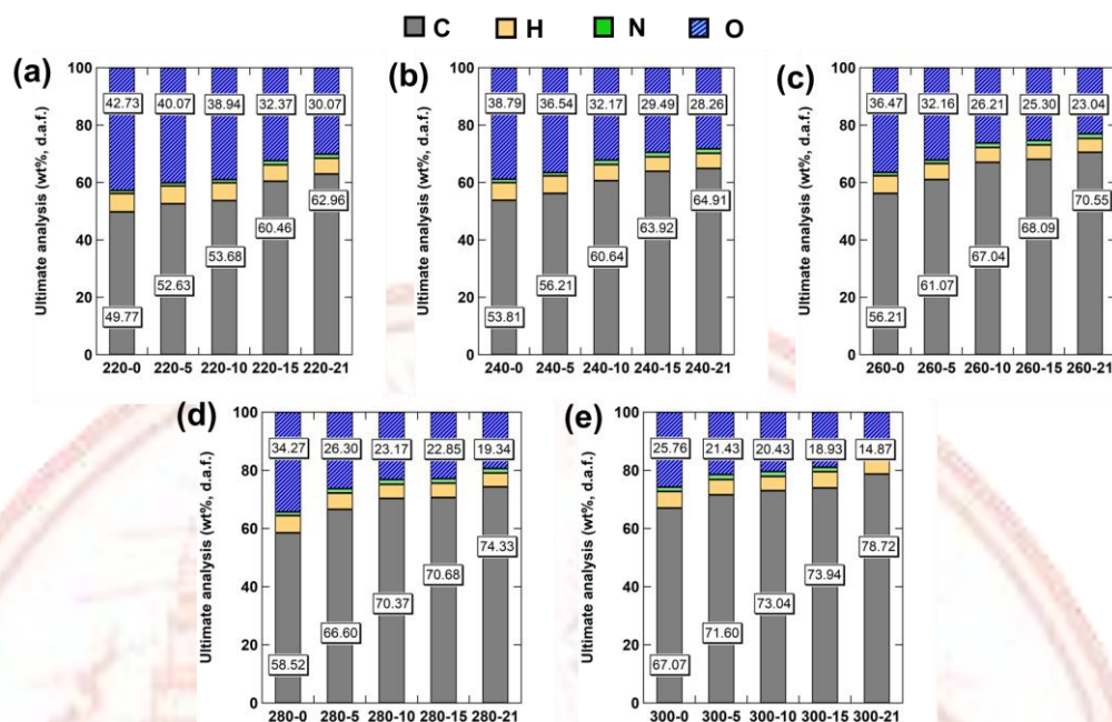
ภาพที่ 4-4 ปริมาณองค์ประกอบของผลิตภัณฑ์ทอร์รีไฟด์เปลือกทุเรียนที่อุณหภูมิ (a) 220 °C (b) 240 °C (c) 260 °C (d) 280 °C และ (e) 300 °C ระยะเวลาที่คงอยู่ในเครื่องปฏิกรณ์ 30 นาที ภายใต้สภาวะออกซิเจนต่างๆ
