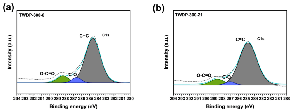
ภาพที่ 4-25 สเปกตรัม XPS ของผลิตภัณฑ์ทอร์รีไฟด์เปลือกทุเรียนในย่านพลังงานของ C1s
