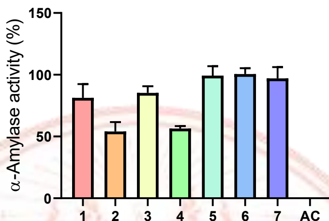
ภาพที่ 4-25ฤทธิ์การต้านเอนไซม์แอลฟาอะไมเลสของสารที่ 1-7
