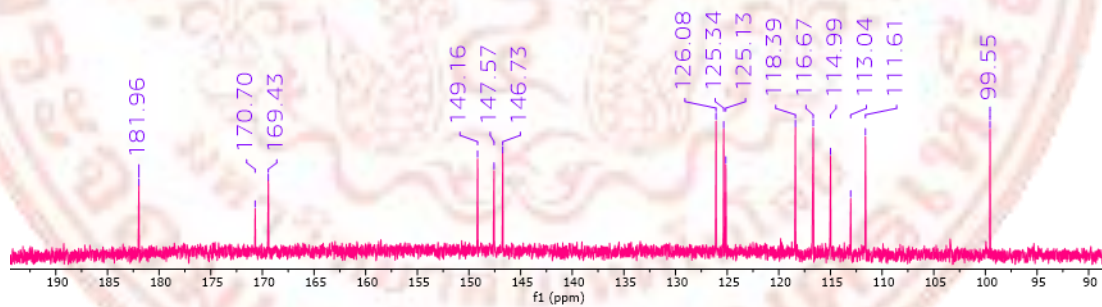
ภาพที่ ก-7 ^{13}\text{C} -NMR (100 MHz, \text{CDCl}_3 ) spectrum ของสาร Sulfuretin (2)
