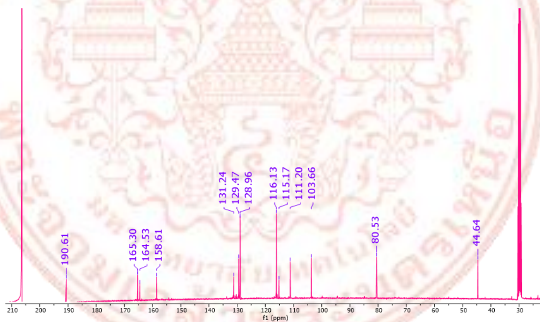
ภาพที่ ก-9 13 C-NMR (100 MHz, Acetone-d 6 ) spectrum ของสาร Liquiritigenin (3)
