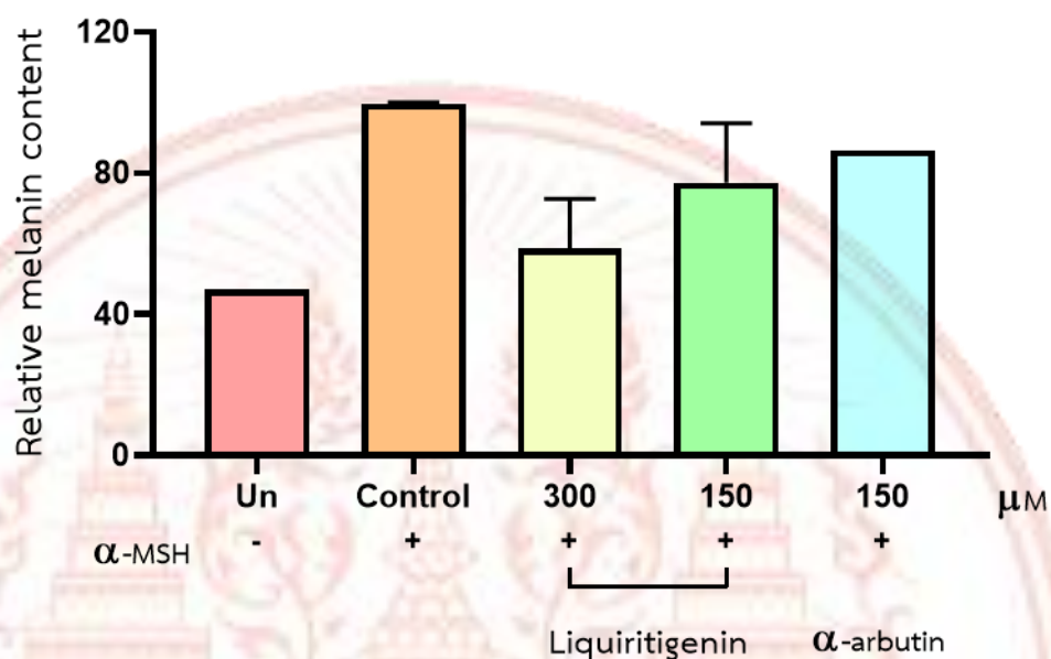
ภาพที่ 4-19 การลดลงของเม็ดสีเมลานินในเซลล์เม็ดสี MNT-1 ของสาร 3
