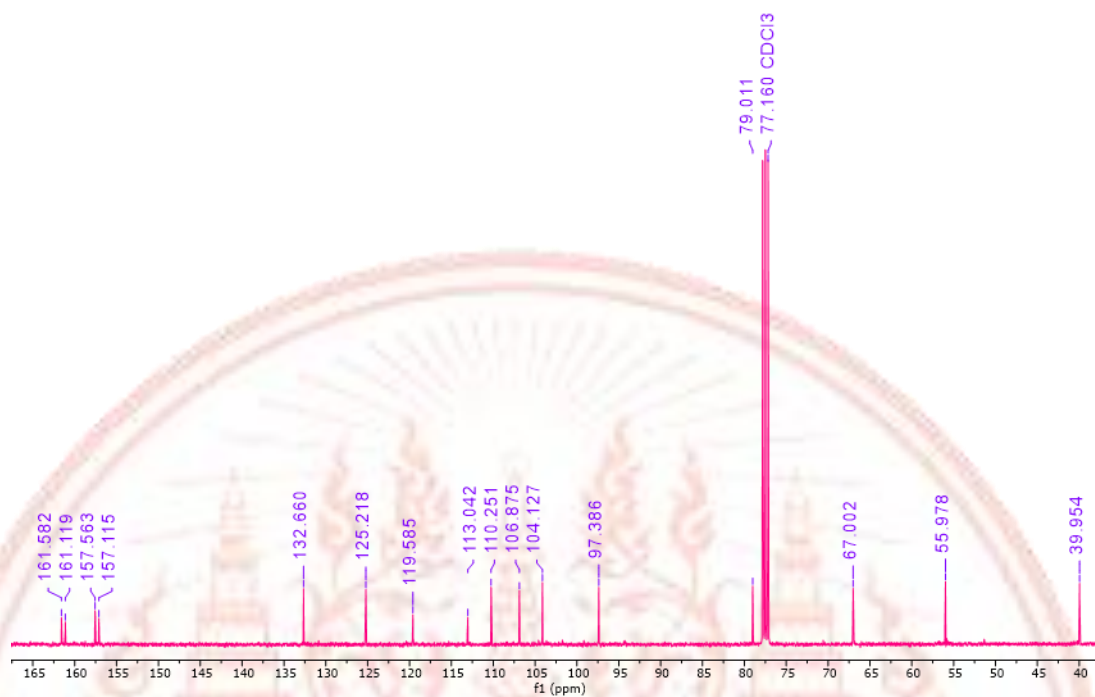
ภาพที่ ก-2 13 C-NMR (100 MHz, CDCl 3 ) spectrum ของสาร Medicarpin (1)
