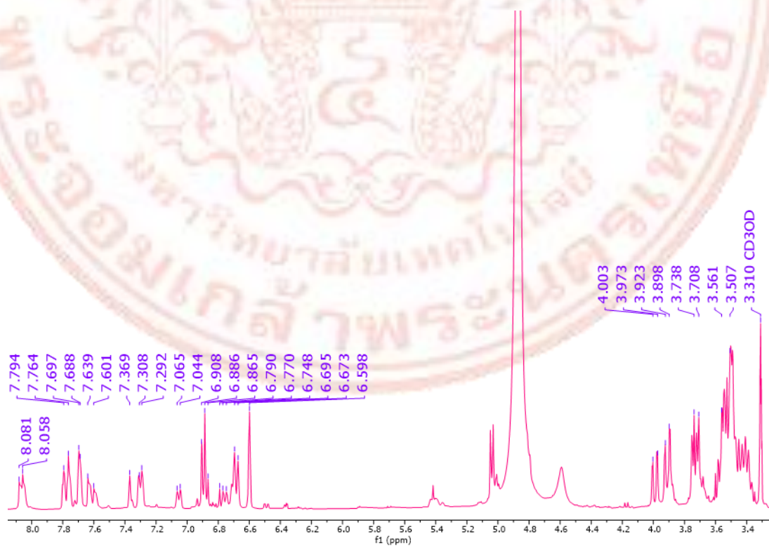
ภาพที่ ก-14 ^1\text{H} -NMR spectrum (400 MHz, \text{CD}_3\text{OD} ) ของสาร Iso-butrin (6)
