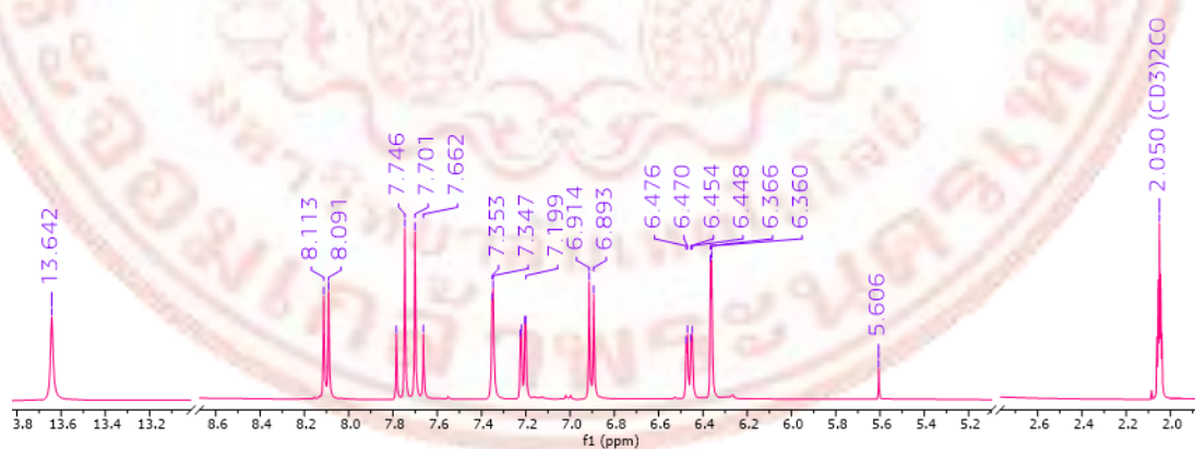
ภาพที่ ก-12 1 H-NMR spectrum (400 MHz, Acetone-d 6 ) ของสาร Butein (5)
