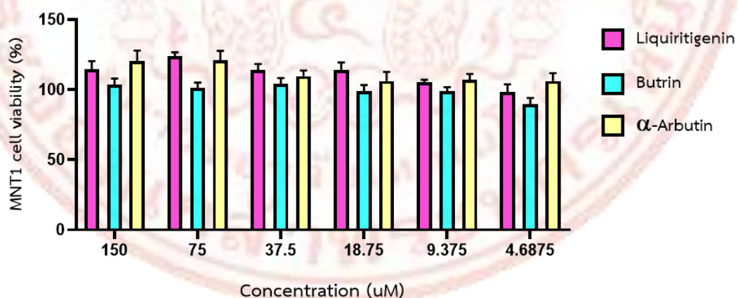
ภาพที่ 4-20 การรอดชีวิตของเซลล์เม็ดสีเมลานโนไซต์ (MNT-1)
