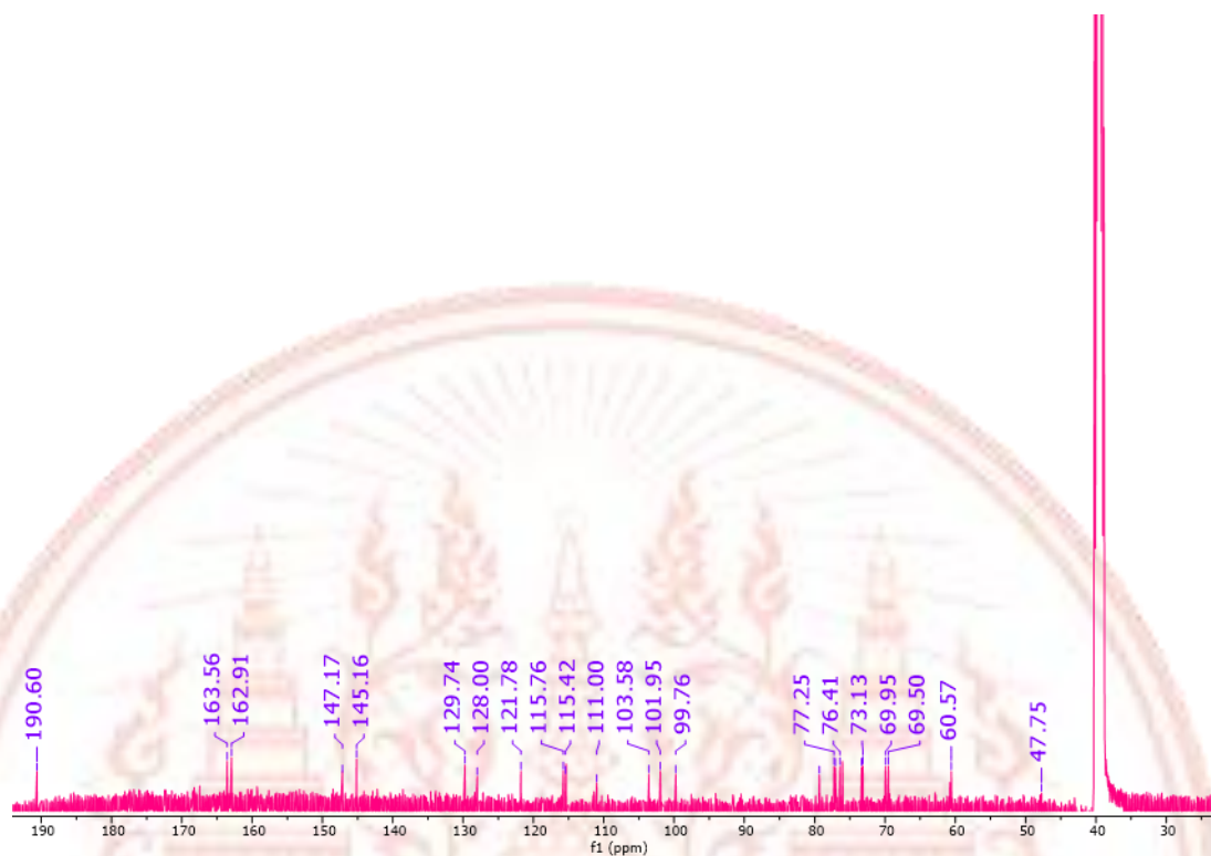
ภาพที่ ก-17 ^{13}\text{C} -NMR (100 MHz, \text{DMSO-d}_6 ) spectrum ของสาร Butrin (7)
