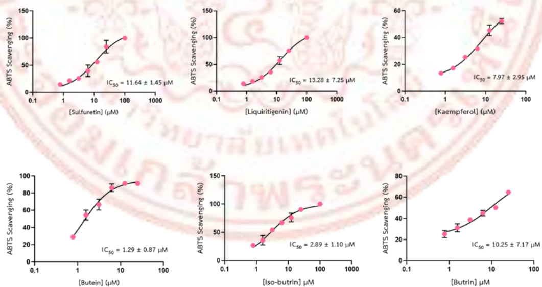
ภาพที่ ก-18 \text{IC}_{50} ของสารประกอบ 2-7 ในการทดสอบฤทธิ์ต้านอนุมูลอิสระด้วยวิธี ABTS
