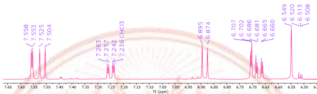
ภาพที่ ก-6 ^1\text{H} -NMR spectrum (400 MHz, \text{CDCl}_3 ) ของสาร Sulfuretin (2)
