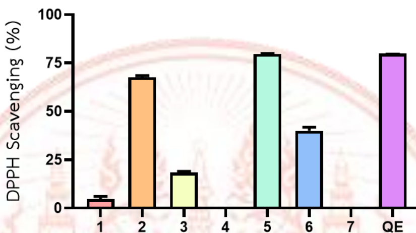
ภาพที่ 4-9ฤทธิ์ในการต้านอนุมูลอิสระด้วยวิธี DPPH ของสาร 1-7
