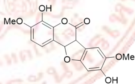
B32 Buteaspermin B
