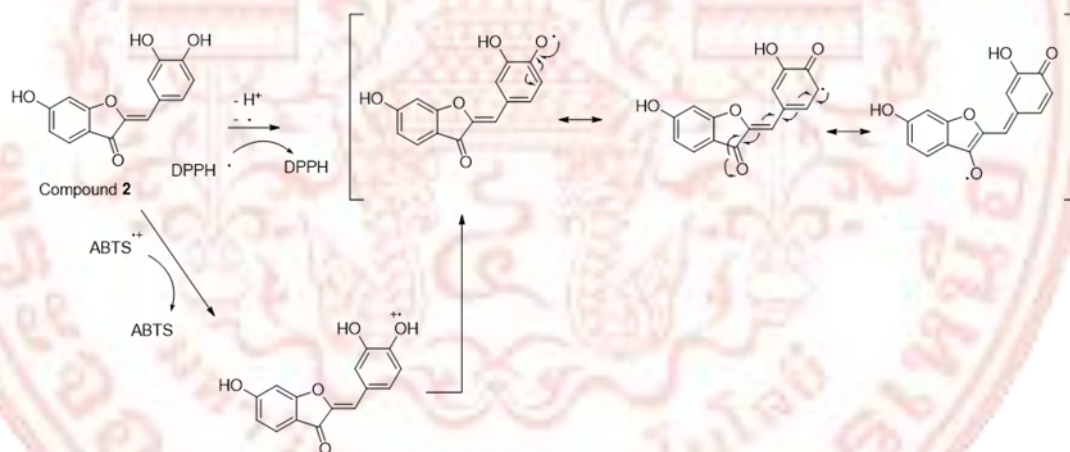
ภาพที่ 4-12 กลไกการยับยั้งอนุมูลอิสระ DPPH• และ ABTS •+ ของสาร sulfuretin (2)
