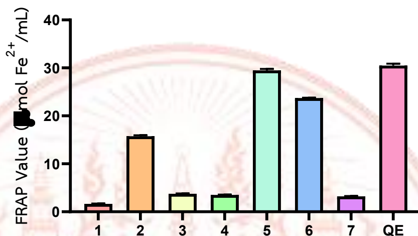
ภาพที่ 4-11 ฤทธิ์ในการต้านอนุมูลอิสระด้วยวิธี FRAP ของสารที่ 1-7
