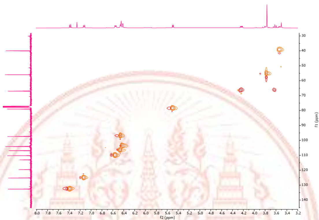
ภาพที่ ก-4 HSQC spectrum ของสาร Medicarpin (1)
