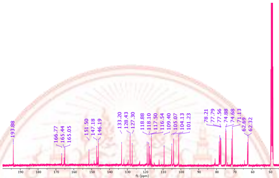
ภาพที่ ก-15 ^{13}\text{C} -NMR (100 MHz, \text{CD}_3\text{OD} ) spectrum ของ Iso-butrin (6)
