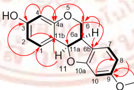
ภาพที่ 4-2 ความสัมพันธ์ HMBC และ ^1\text{H} - ^1\text{H} COSY ของสาร Medicarpin (1)
