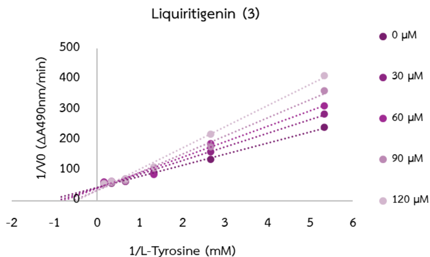
ภาพที่ 4-17 กราฟ Lineweaver-Burk แสดงการยับยั้งการทำงานของเอนไซม์ไทโรซิเนส โดยสาร liquiritigenin ในช่วงความเข้มข้น 30–120 \mu\text{M} โดยใช้ L-tyrosine เป็นซับสเตรตในช่วงความเข้มข้น 0.15–4.8 mM
