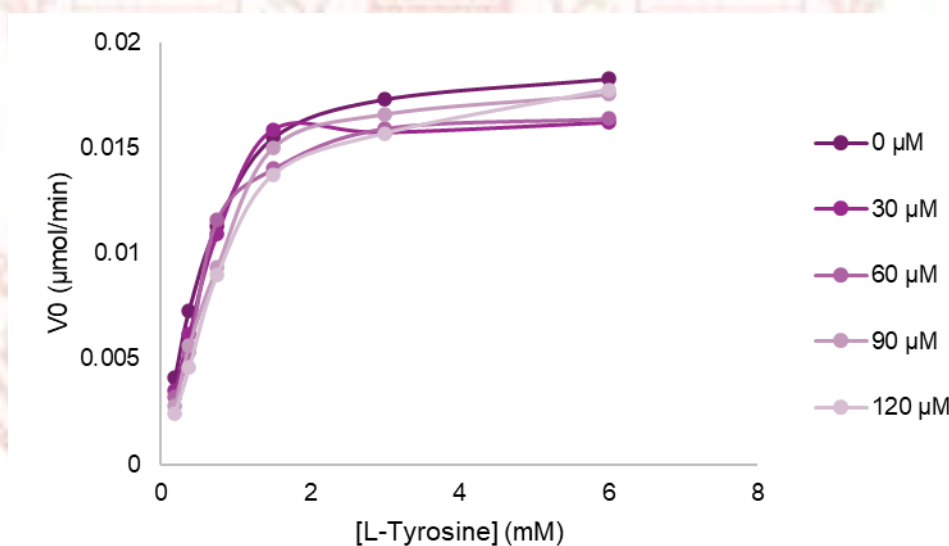
ภาพที่ 4-16 กราฟ Michaelis-Menten ของสาร 3
