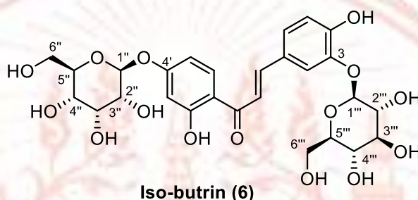
ภาพที่ 4-7 โครงสร้างสารที่ 6
