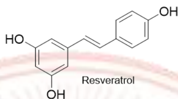
ภาพที่ 2-2 โครงสร้างทางเคมีของสารประกอบสตีลบิน
