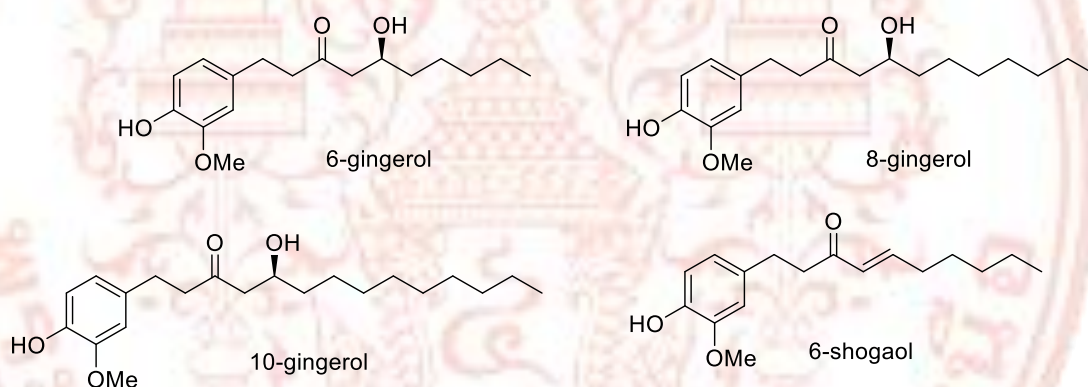
ภาพที่ 2-4 โครงสร้างทางเคมีของสารประกอบที่พบในจิง
