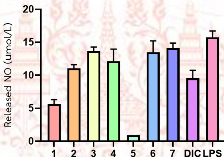
ภาพที่ 4-21 ปริมาณไนตริกออกไซด์ (NO) ที่ถูกปล่อยออกมาโดยใช้สารที่ความเข้มข้น 150 \mu\text{M}
