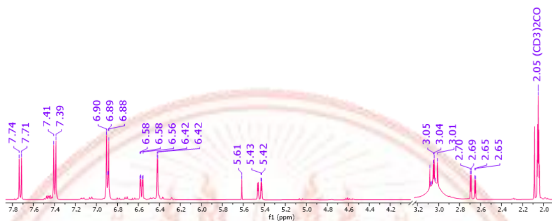
ภาพที่ ก-8 1 H-NMR spectrum (400 MHz, Acetone-d 6 ) ของสาร Liquiritigenin (3)
