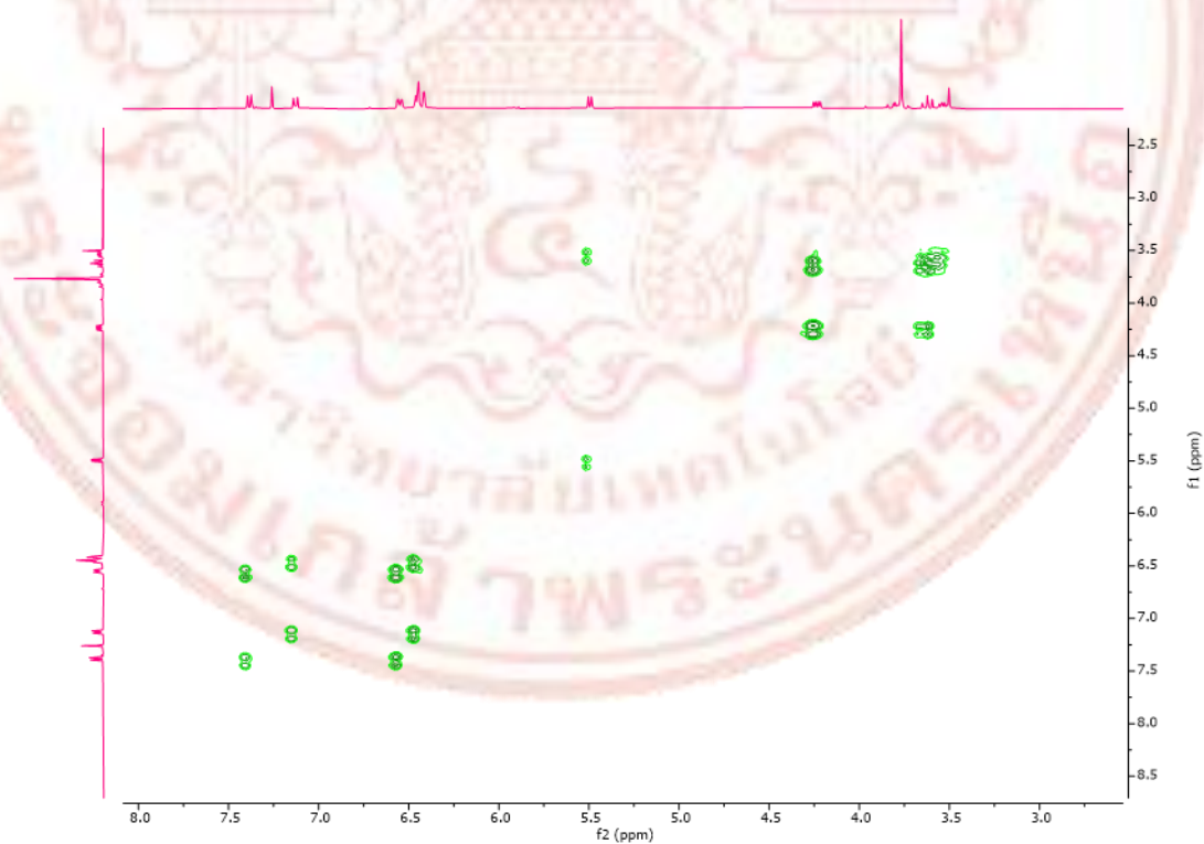
ภาพที่ ก-3 COSY spectrum ของสาร Medicarpin (1)
