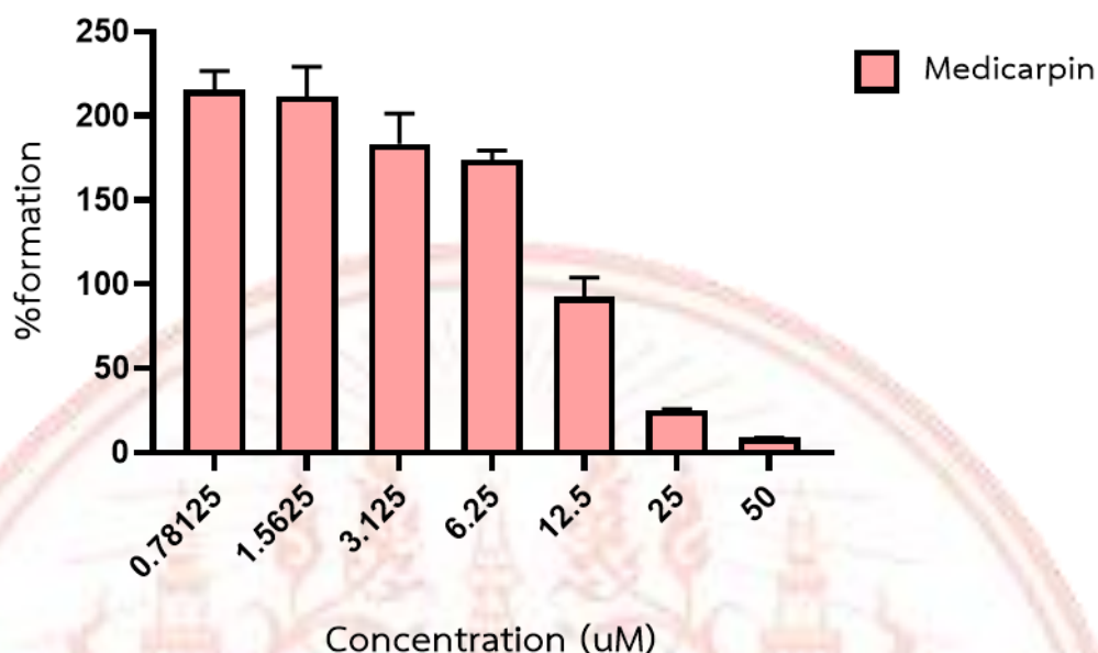
ภาพที่ 4-24 การก่อตัวไบโอฟิล์มของแบคทีเรีย S. aureus ATCC 10832 ของสาร medicarpin (1)
