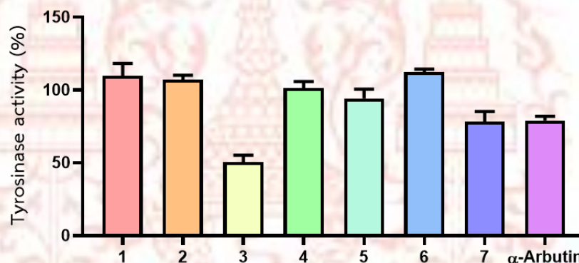
ภาพที่ 4-13 ฤทธิ์ในการต้านเอนไซม์ไทโรซิเนสของสารที่ 1-7
