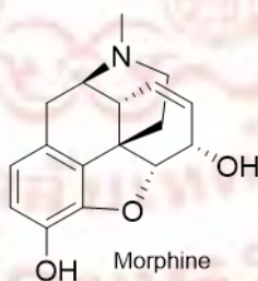
ภาพที่ 2-1 โครงสร้างทางเคมีของสารประกอบแอลคาลอยด์
