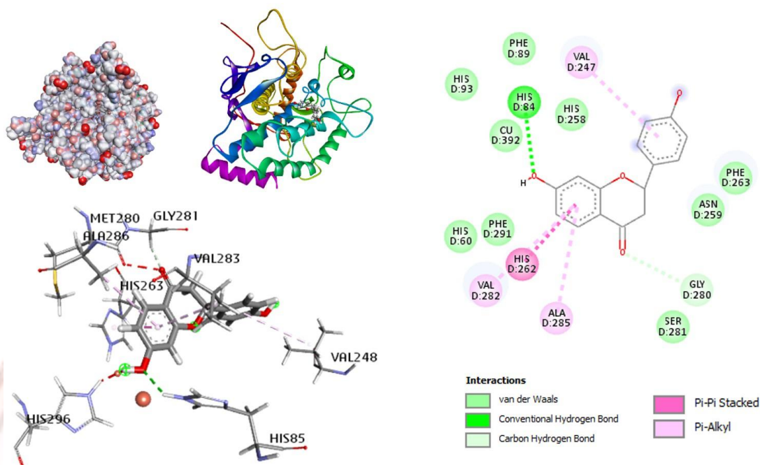
ภาพที่ 4-15 อันตรกิริยาของ liquiritigenin (3) ภายในบริเวณเร่งของเอนไซม์ไทโรซิเนส
