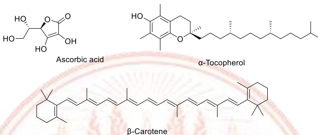
ภาพที่ 2-3 โครงสร้างทางเคมีของ 3 สารต้านอนุมูลอิสระ (Antioxidants)
