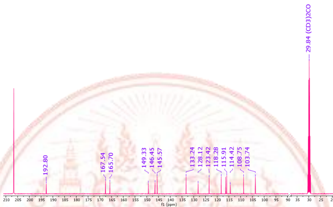
ภาพที่ ก-13 ^{13}\text{C} -NMR (100 MHz, Acetone- \text{d}_6 ) spectrum ของสาร Butein (5)
