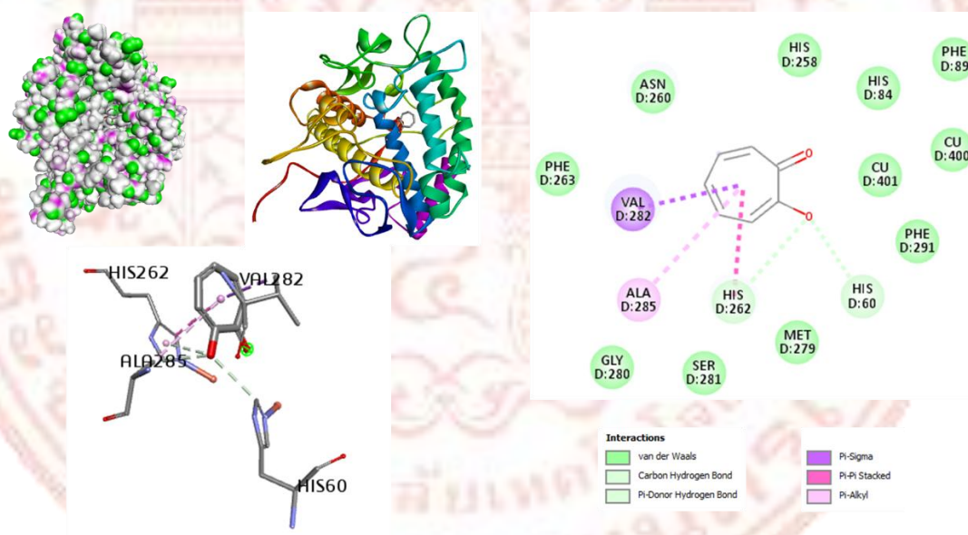
ภาพที่ 4-14 อันตรกิริยาของ Tropolone ภายในบริเวณเร่งของเอนไซม์ไทโรซีนเนส
