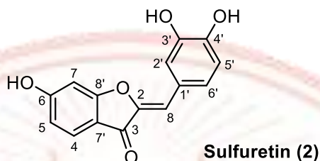
ภาพที่ 4-3 โครงสร้างสารที่ 2
