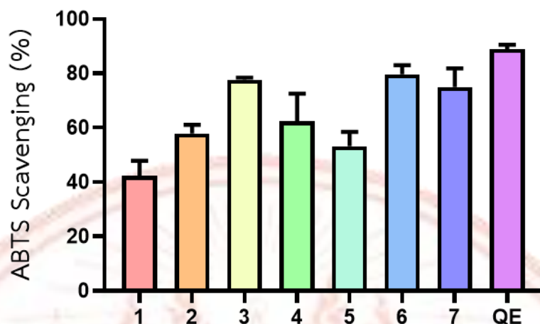
ภาพที่ 4-10 กิจกรรมการต้านอนุมูลอิสระ ABTS ของสารที่ 1-7
